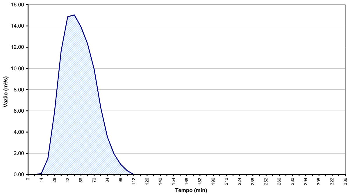
Figura 5.4 - Hidrograma definitivo
